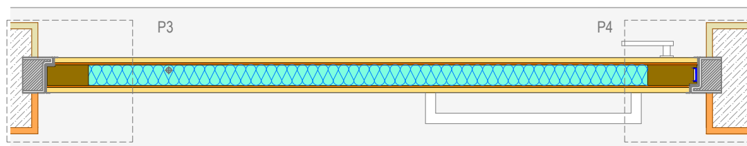
corte horizontal esc 1/10
