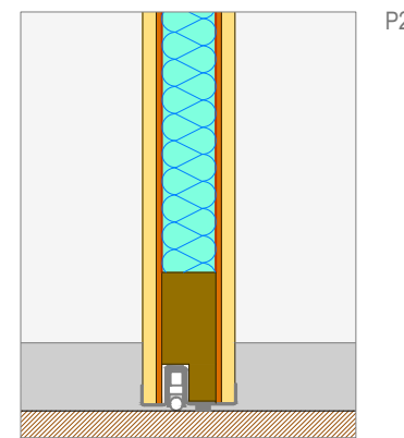
corte vertical esc 1/5
