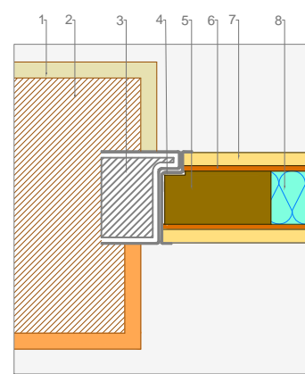
corte horizontal esc 1/5
