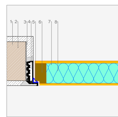
corte horizontal esc 1/5
