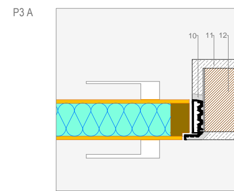
corte horizontal esc 1/5
