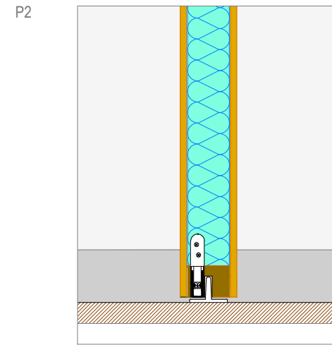
corte vertical esc 1/5
