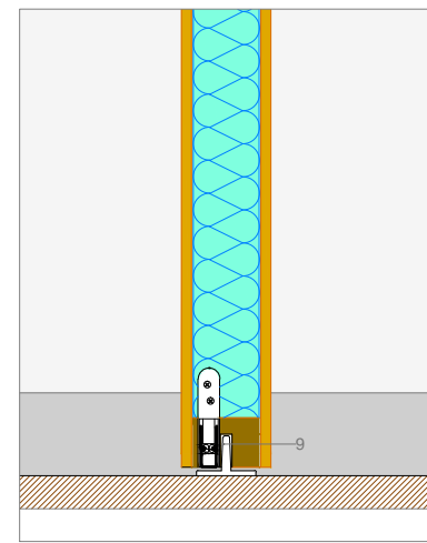
corte vertical esc 1/5
