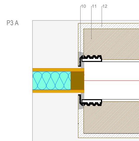
corte horizontal esc 1/5
