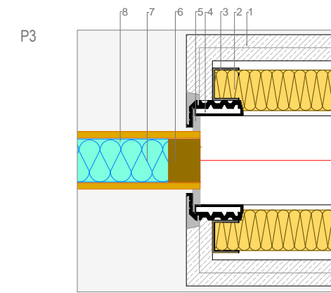
corte horizontal esc 1/5
