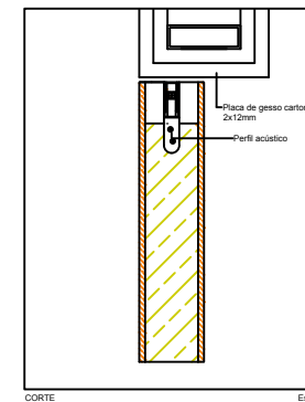
CORTE Esc. 1/5
